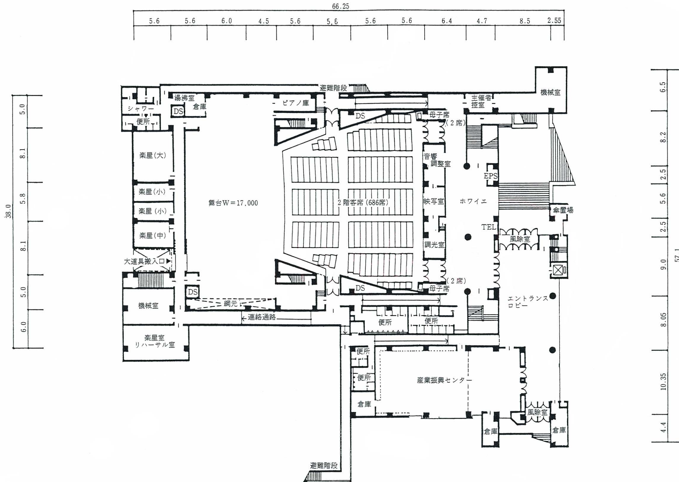
2階平面図 (S. 1/400)
